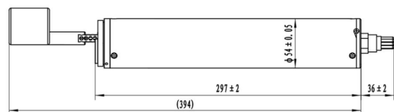
DW1613-D 直读自容一体式温盐深仪 - 6000m
