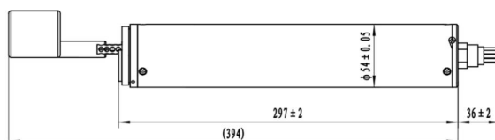
DW1623-D 直读式温盐深仪 - 6000m
