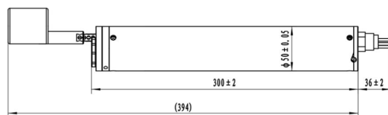
DW1623 直读式温盐深仪 - 1500m
