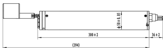
DW1613 直读自容一体式温盐深仪 - 1500m
